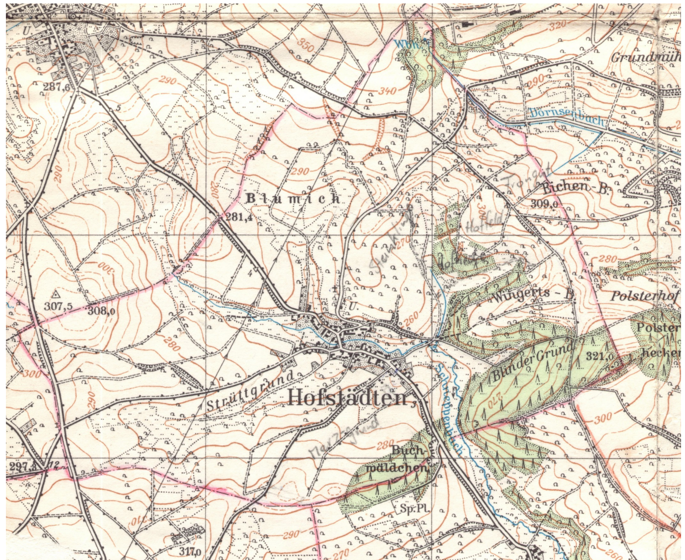
Ausschnitt aus dem Meßtischblatt von 1963
